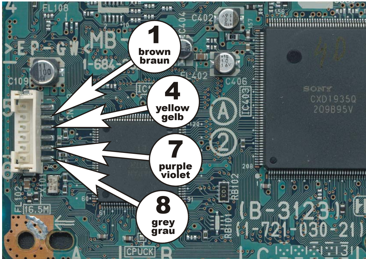
Mainboard (top side) NS305
